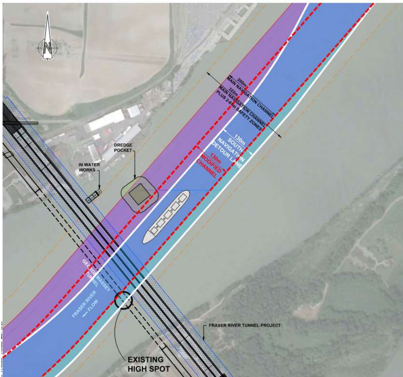
SITE PLAN 1:3000
